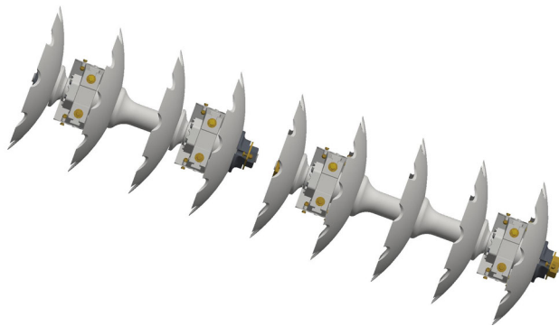
GPCR 18 discos 6 mancais DMO 8 separadores
