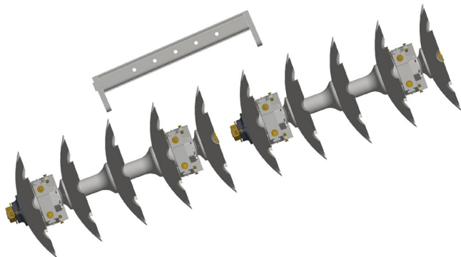
GPCR 20 discos 8 mancais DMO 8 separadores
